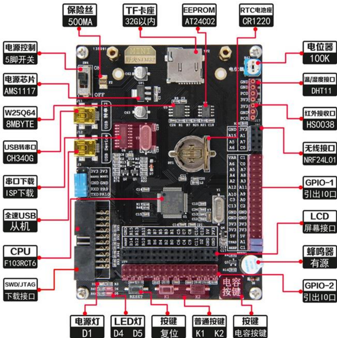
图 2.3-1 开发板硬件资源图
