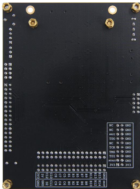
图 2.1-3 MINI 开发板背面视图
