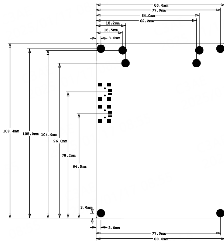
图 2.2-1 MINI 开发板机械尺寸图
