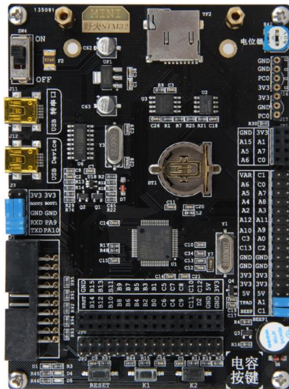
图 2.1-1 MINI 开发板正面视图
